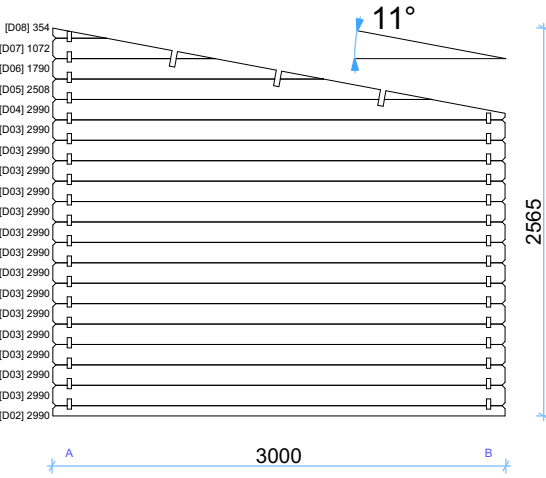
Wall D 1:50
